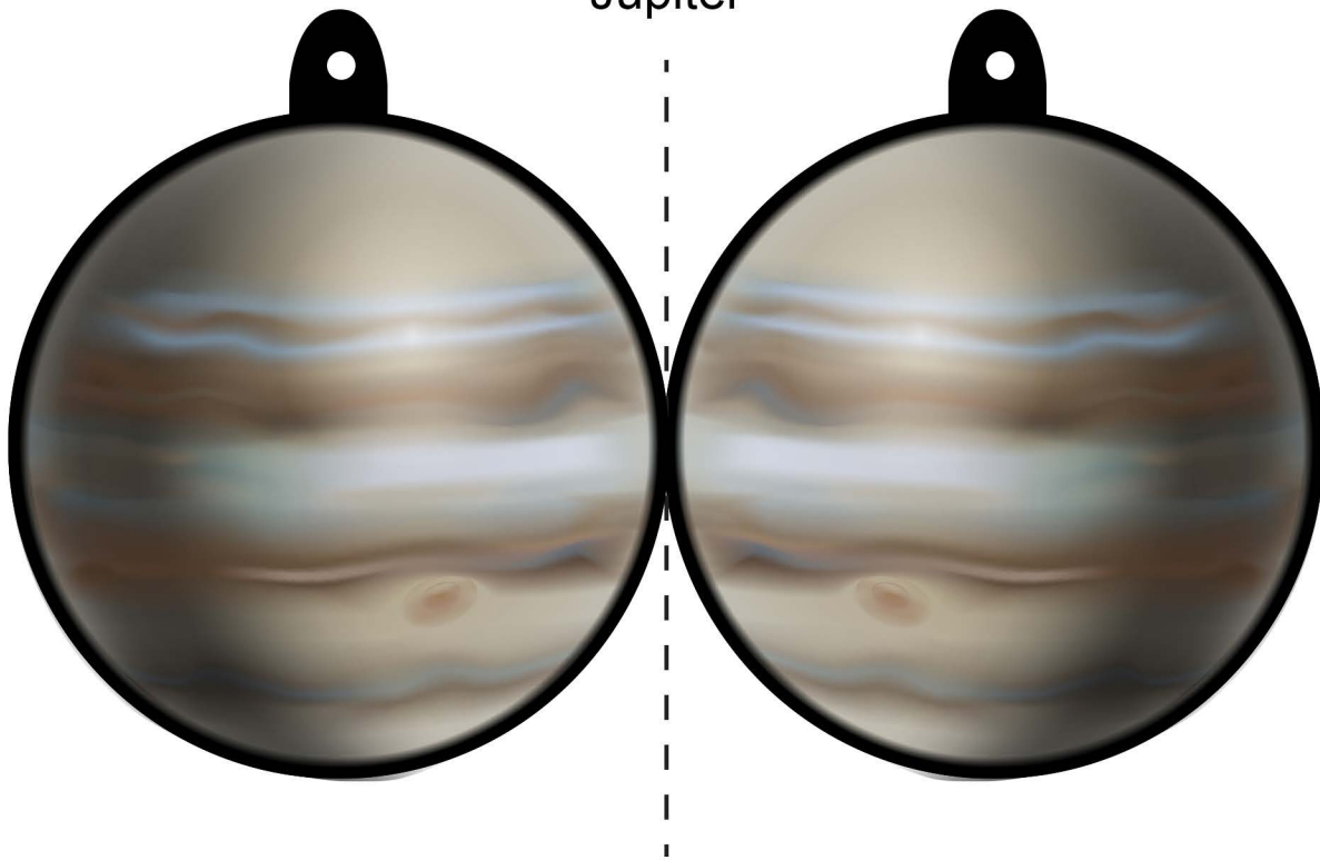
Jupiter
