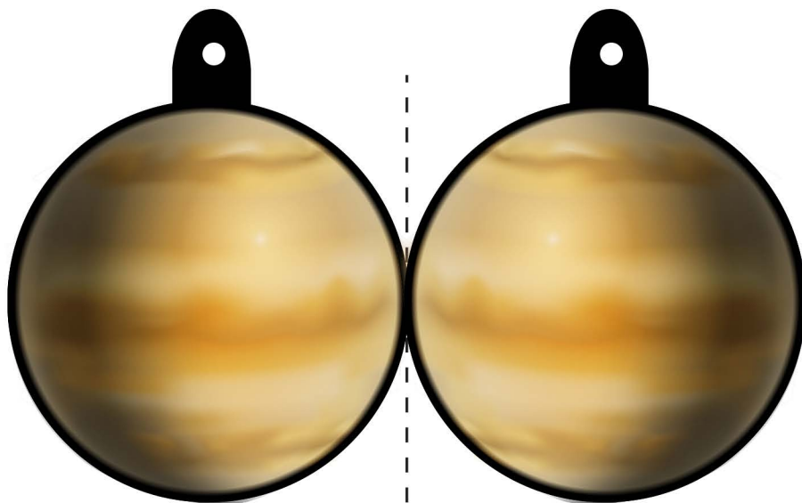
Venus
