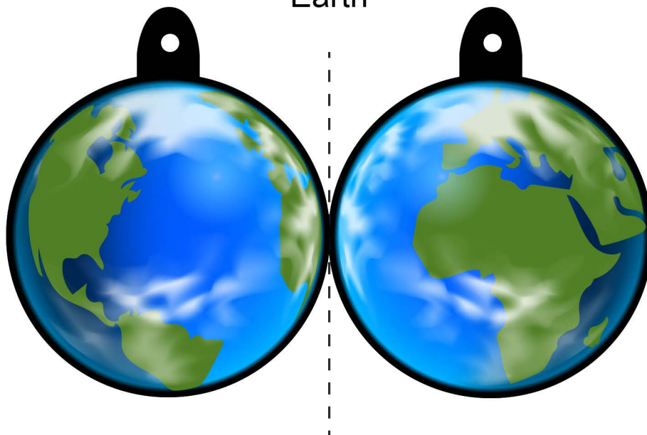
Earth
