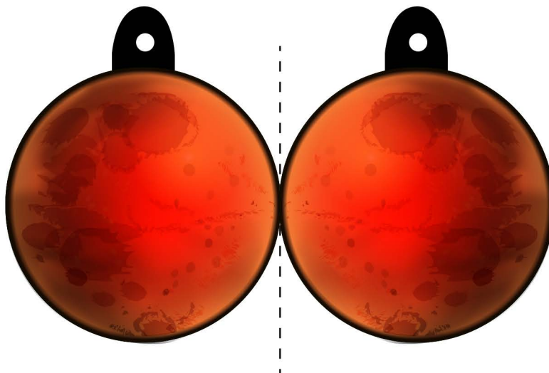
Mars
