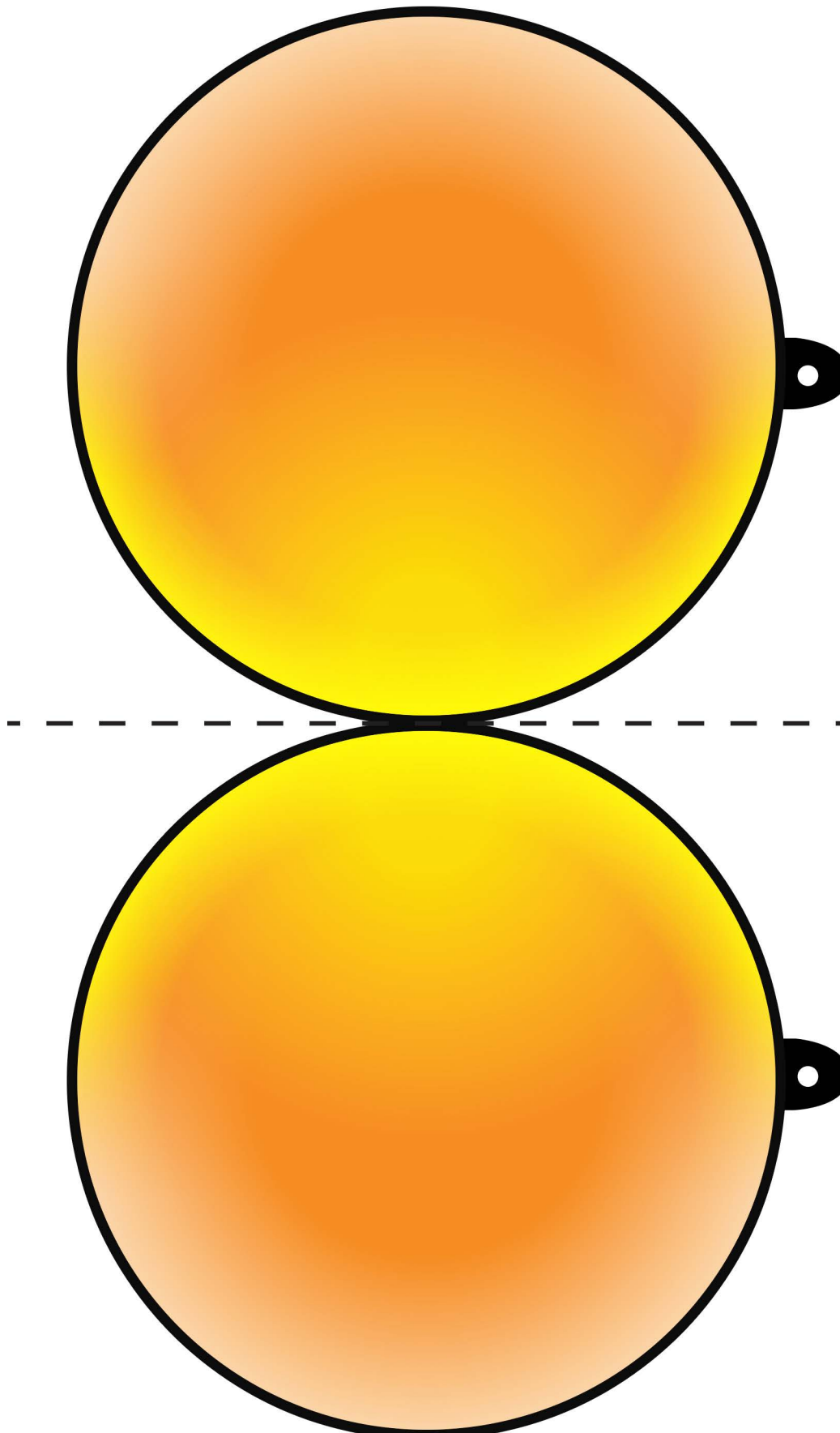
Sun
